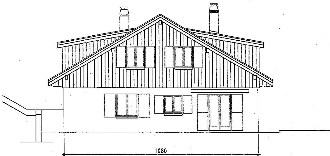
FACADE SUD-OUEST
